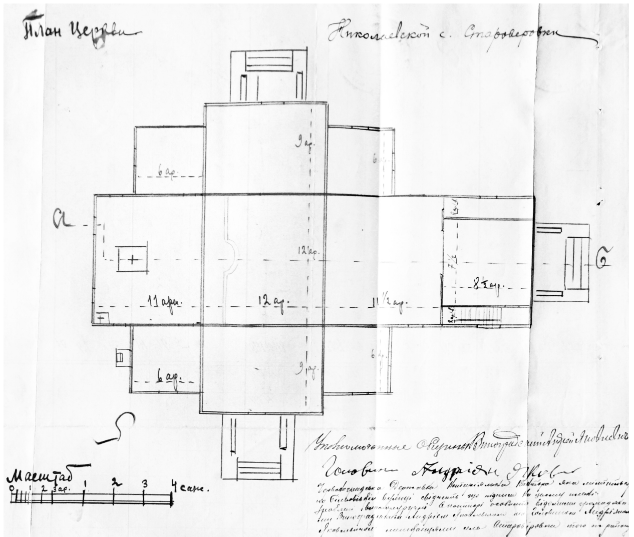
План Николаевской церкви, 1925 год
