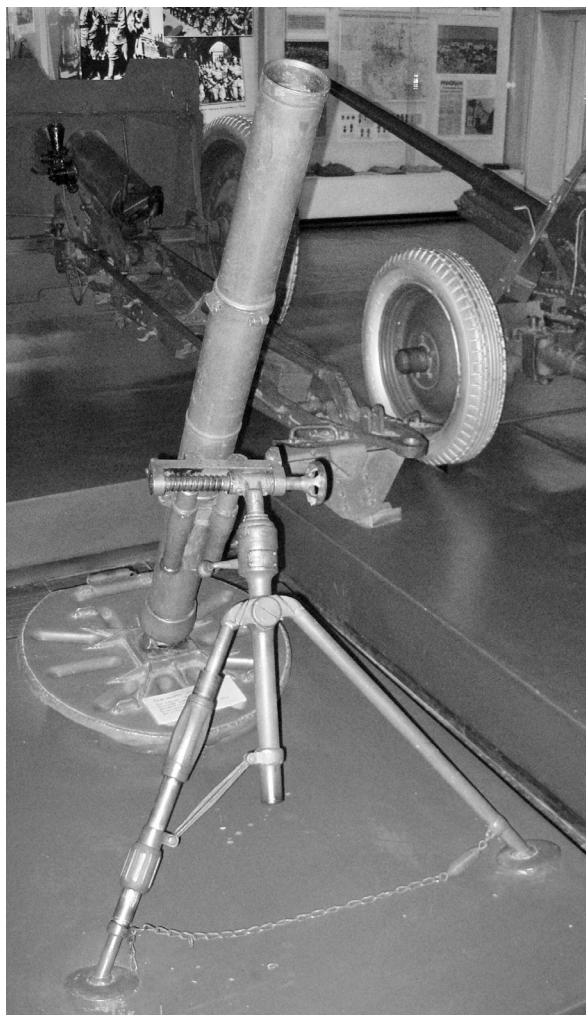
82-мм миномет образца 1937 г.
