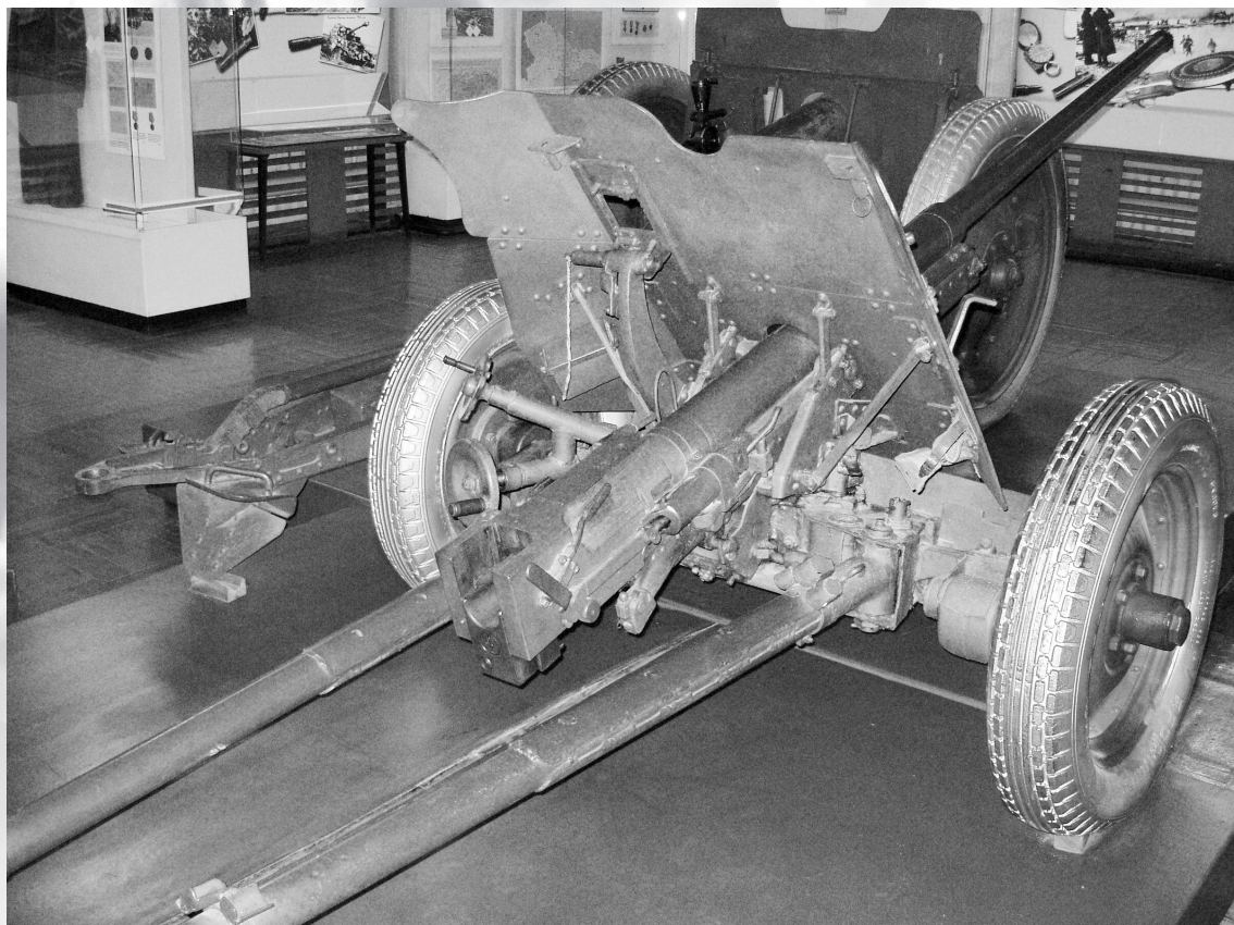
45-мм противотанковая пушка образца 1942 г.
