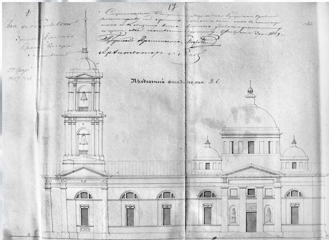
Проект Архангело-Михайловской церкви в с. Тарановка
